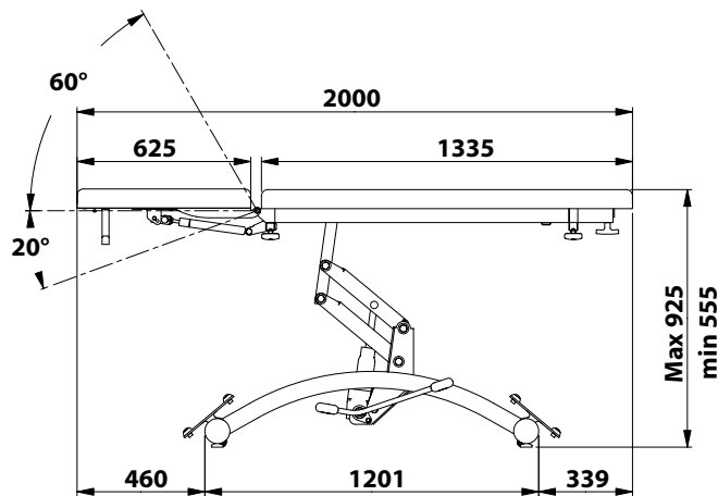
Modèles / Models 1050-10 / 1050-15
